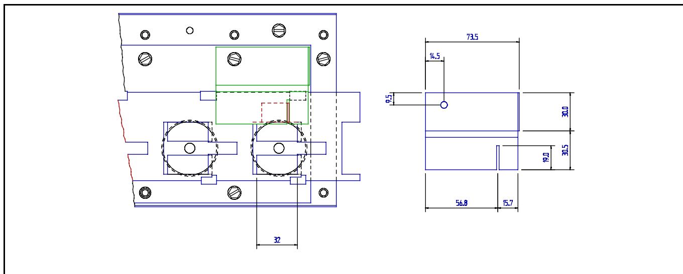
Figuur 8 : Positie luchtschuif
