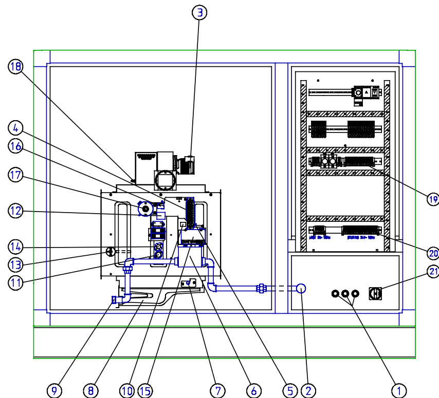
Figuur 9 : Overzicht componenten (afhankelijk van uitvoering)
