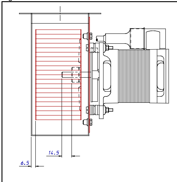
Figuur 6 : Critische maten
