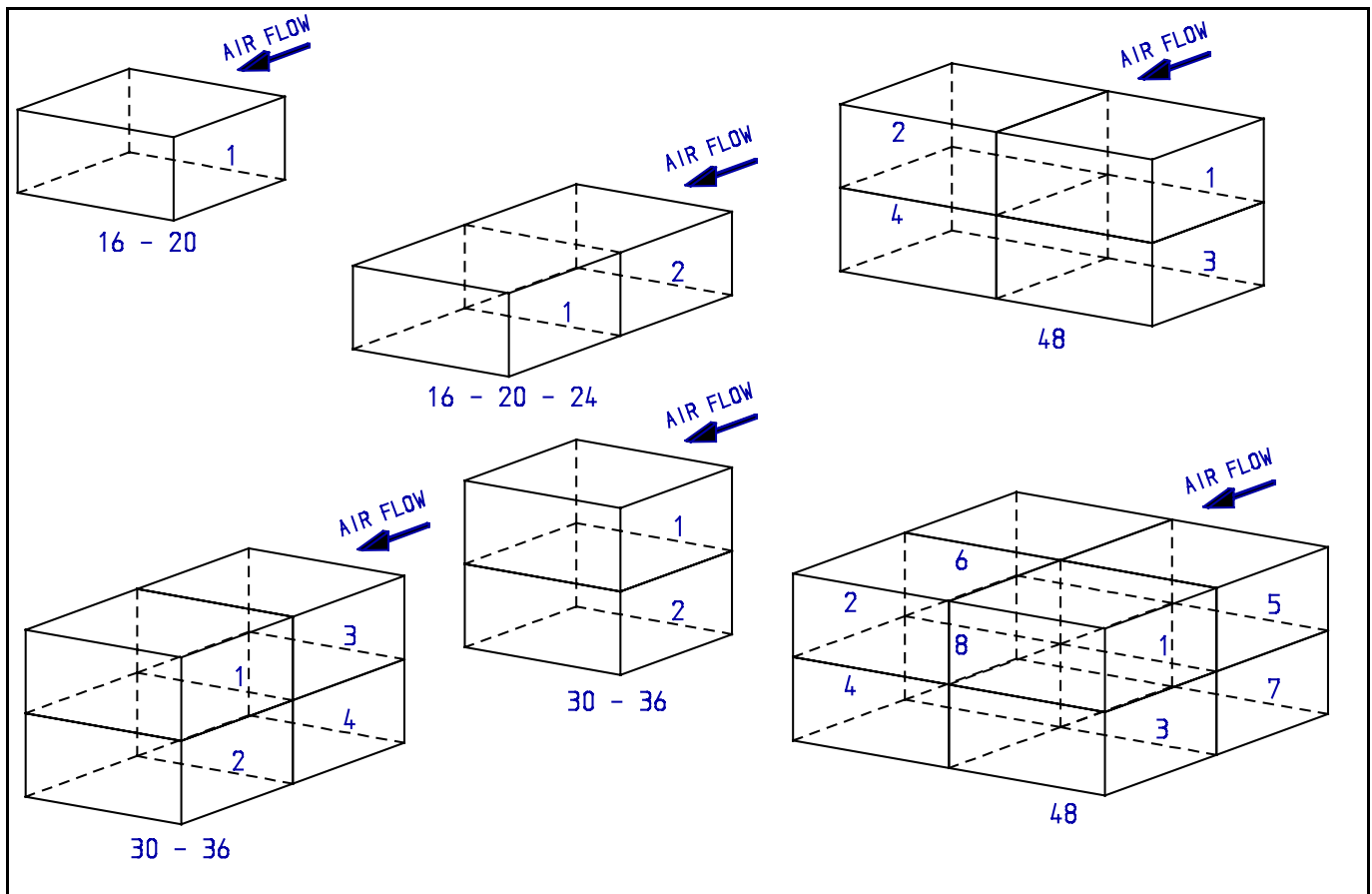
Figuur 2 : Volgorde van het inkomen van de verwarmingssecties bij meertrapsregeling
