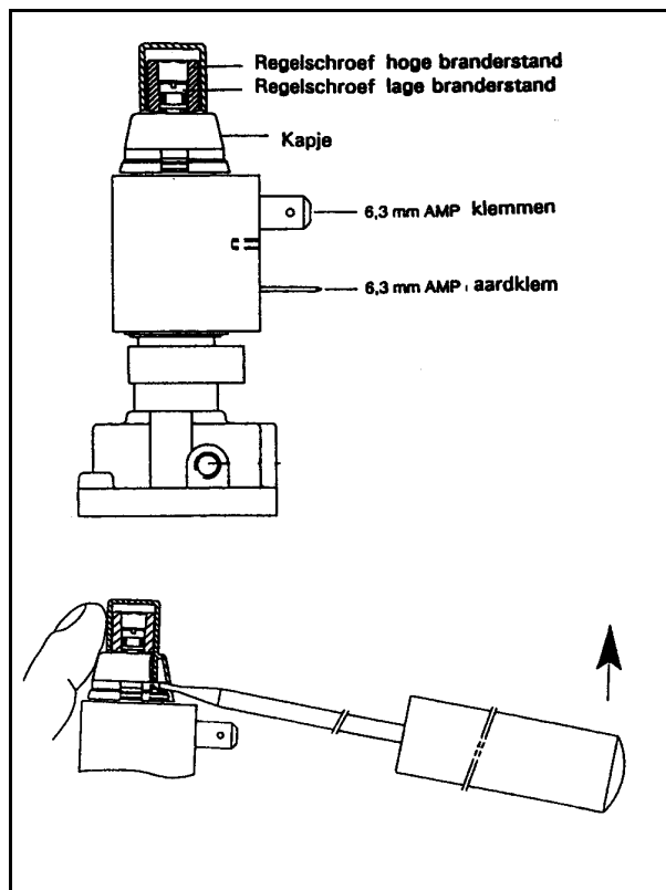
Figuur 3 : Instellen branderdruk
