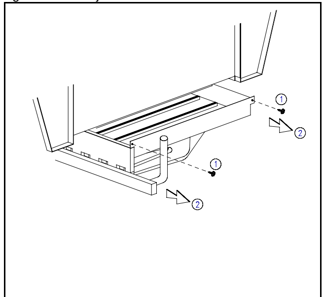
Figuur 7 : verwijderen branderrek
