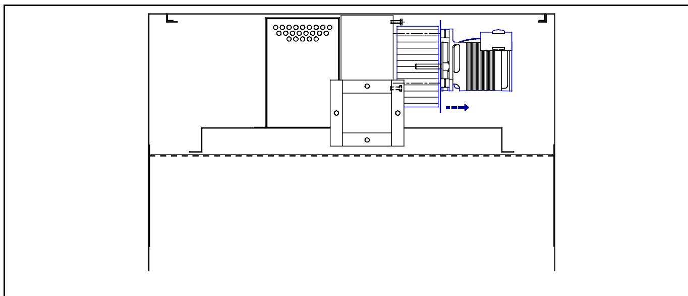
Figuur 5 : Verwijderen van de rookgasventilator
